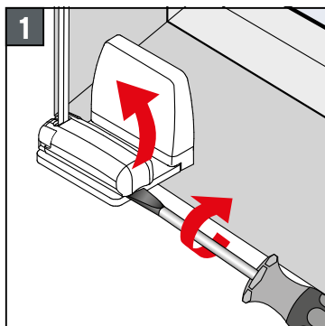
Winkelmontage Face fixing Montage en angle Montaggio ad angolo
