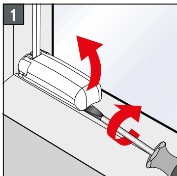
Falzmontage Top fixing Montage en feuillure Montaggio a libro
