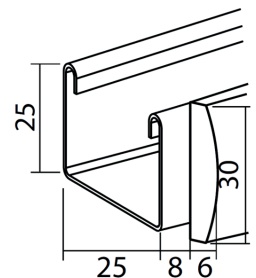
Kopfschiene mit Blende
